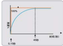
* LED光源对比白色冷阴极射线荧光灯预热时间 * Sharpshot LED光源 * 白色冷阴极射线荧光灯
